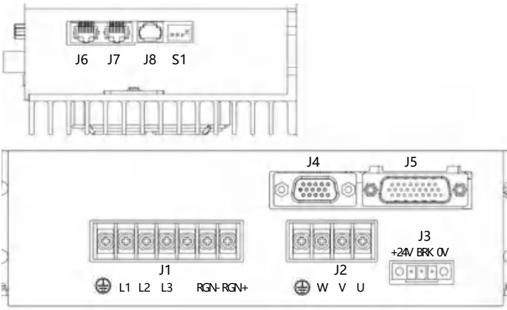
J3 内部24v输出端子
